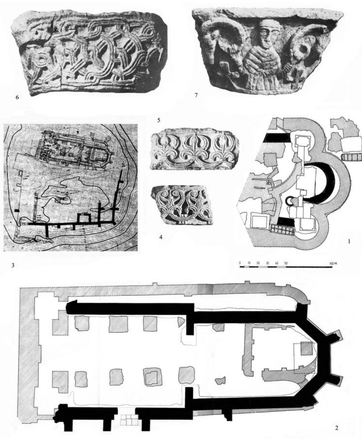
Сл. 79. Најважнији храмови Сремске епископије: 1. Мачванска Митровица, источни део цркве са главним грађевинским фазама из 4-6, 8-10, 11-12. и 13-15. столећа; 2. Раковац (Домбо), задужбина намесника Мађарске Белоша, основа базилике 12. столећа и готичке цркве изнад ње, 3. план манастира, 4-7. греде и капители украшени рељефима.
