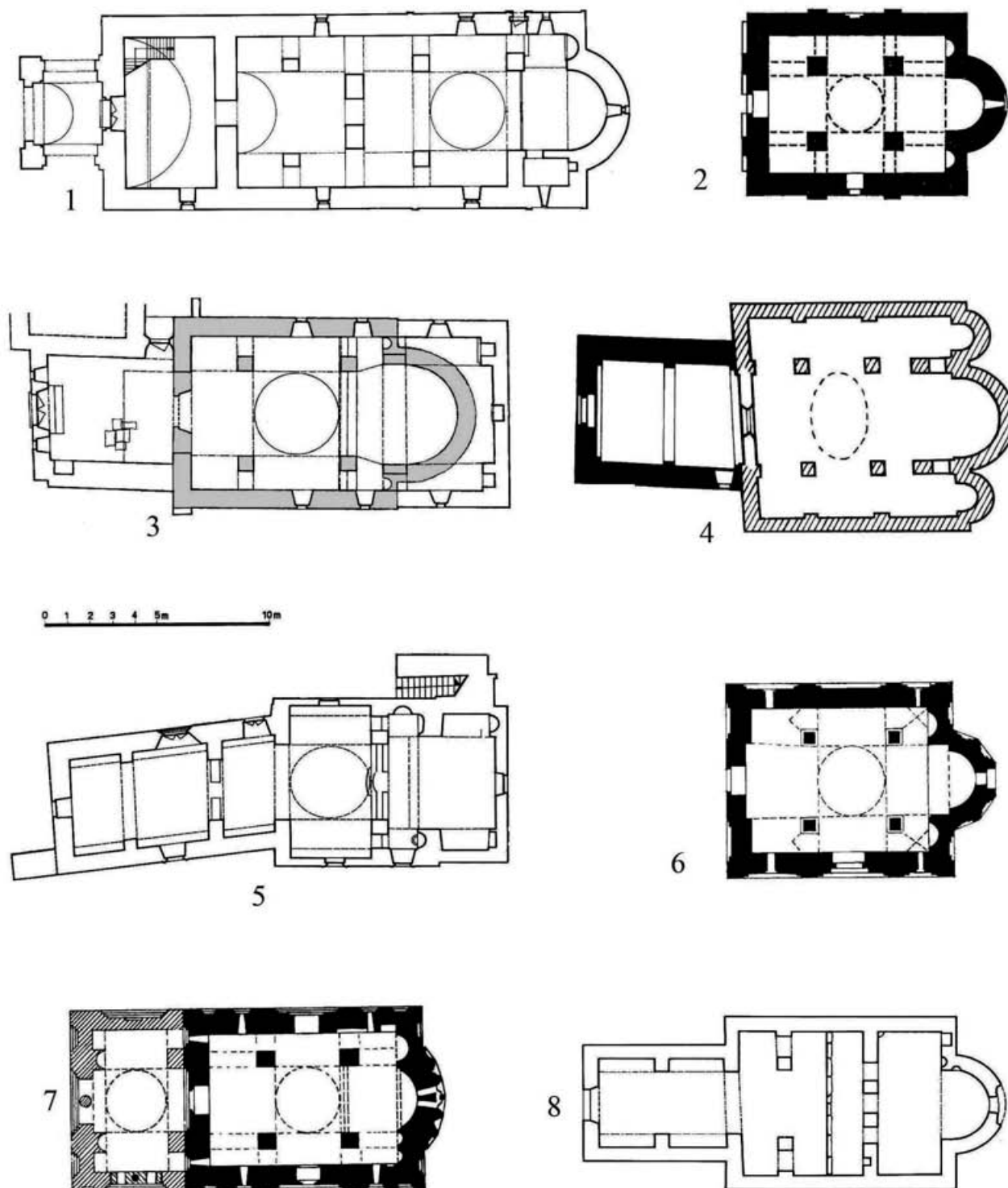
Сл. 86. Основе манастирских цркава на српском западу и сличних на истоку: 1. Гомионица; 2. Муштуиште; 3. Крупа код Зрмање; 4. Тврдош; 5. Крка (неиспитана); 6. Љуботен; 7. Лесново; 8. Рмањ.
